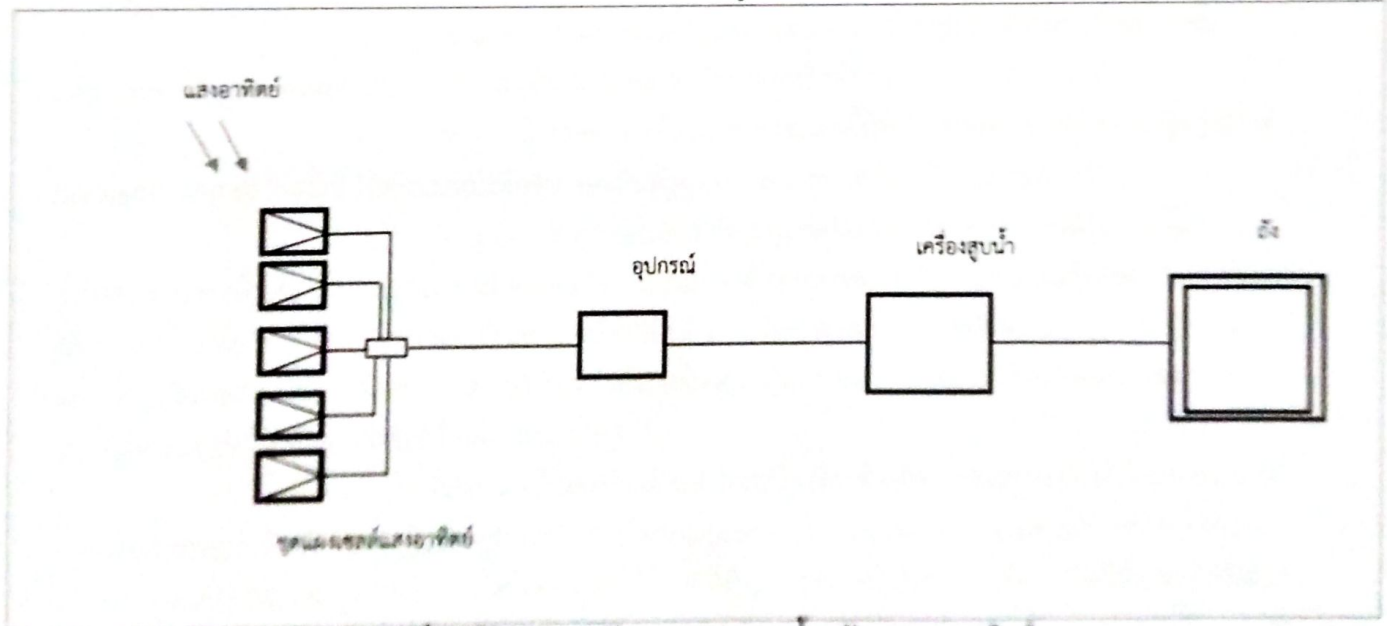
รูปที่ ๑ ไดอะแกรมลักษณะระบบสูบน้ำพลังงานแสงอาทิตย์
